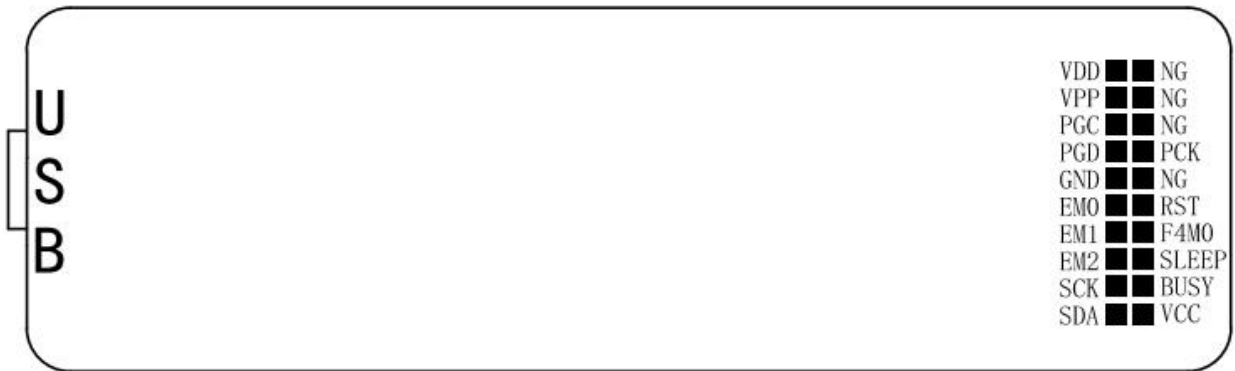
图 2-3 HC-ICDPRO V1.0 主板引脚图
